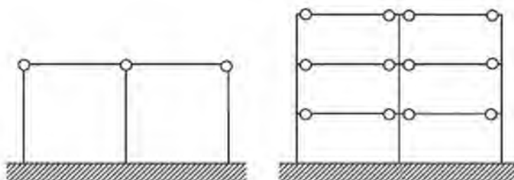
Figura C7.4.5 - Strutture con pilastri incastrati alla base ed orizzontamenti ad assi cernierali
