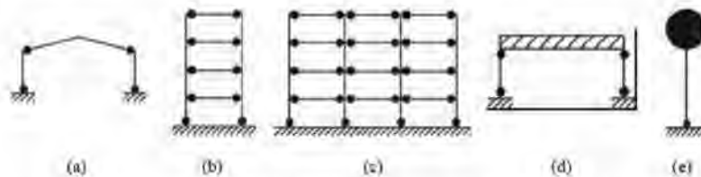
Figura C7.5.1 – Configurazioni dissipative di strutture intelaiate: disposizione delle cerniere plastiche, secondo le tipologie esposte nella Tabella 7.3.11 del § 7.3.1 della NTC.
