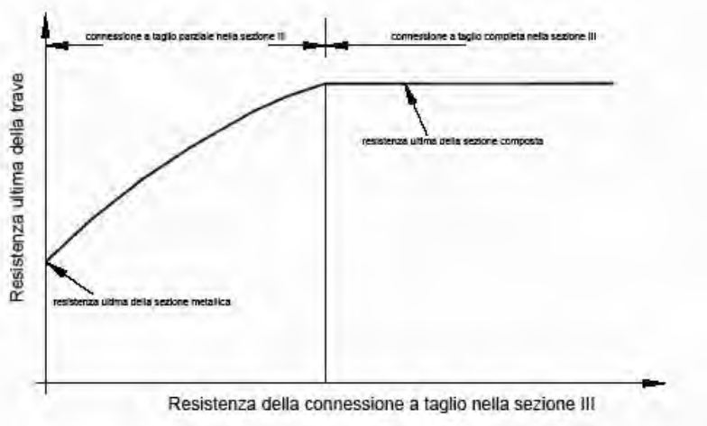
Figura C4.3.5 – Legame tra resistenza della trave e resistenza della connessione
