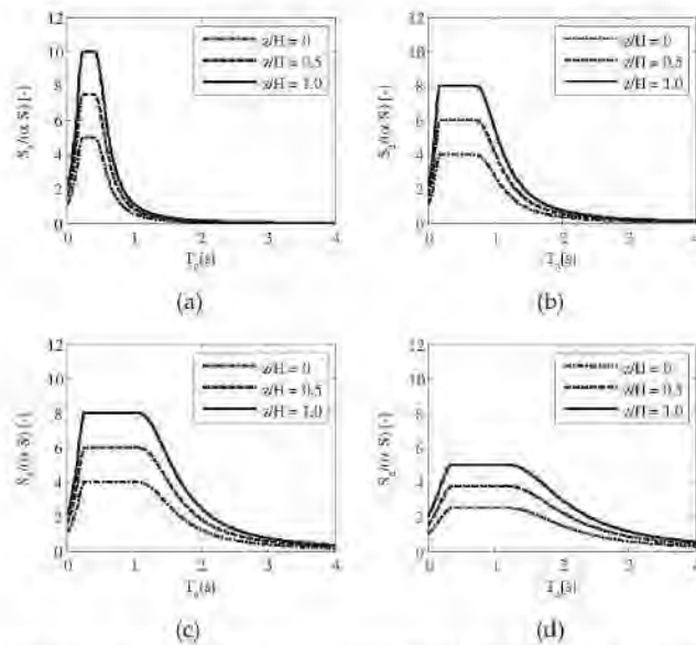
Figura C7.2.4 - Accelerazione massima, normalizzata rispetto ad \alpha S , per i seguenti valori di T_d : (a) T_d = 0,3 s, (b) T_d = 0,6 s, (c) T_d = 0,9 s, (d) T_d = 1,2 s.
