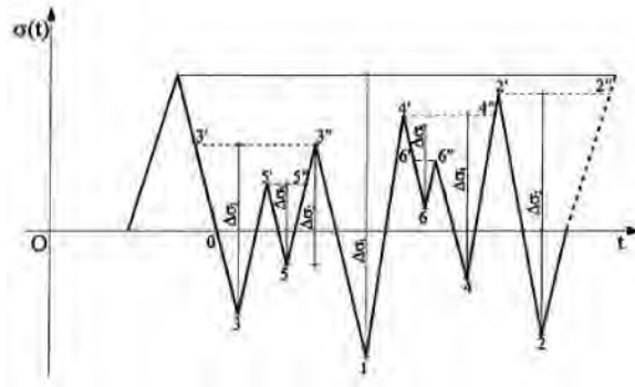
Figura C4.2.19 - Metodo del serbatoio
