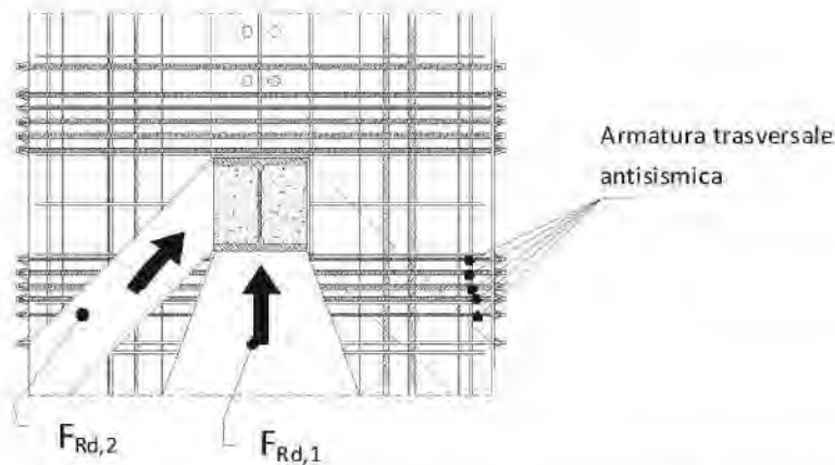
Figura C7.6.3-Vista in pianta dei meccanismi resistenti attuabili nella soletta compressa (momento positivo)
