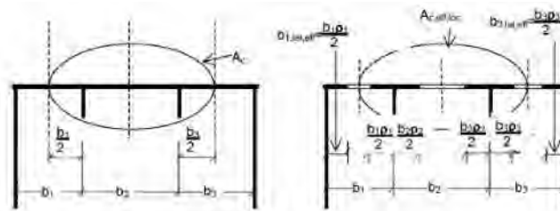
Figura C4.2.15 - Lastra irrigidita uniformemente compressa
