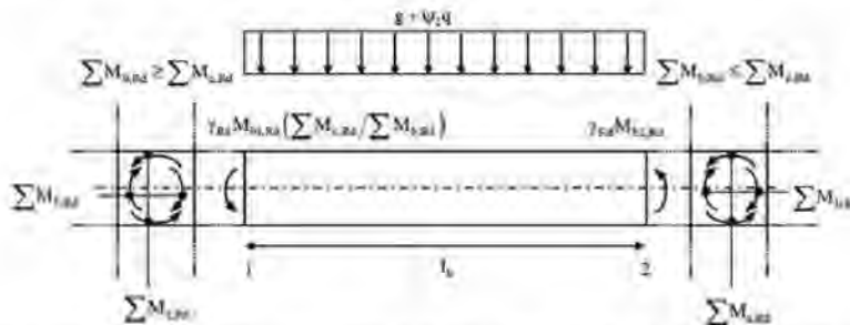
Figura C7.4.1 - Equilibrio dei momenti per il calcolo delle sollecitazioni di taglio di progetto in una trave.
