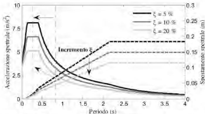
Figura C7.10.2 - Strategia di riduzione della domanda mediante dissipazione di energia
