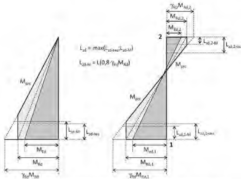
Figura C7.9.1 – Progettazione in capacità delle pile (schiuma mensola e a doppio incastro)
