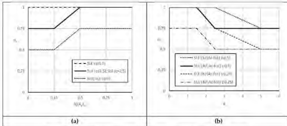
Figura C7.2.5 Dipendenza di \alpha dal carico assiale N e dal fattore di comportamento q .
